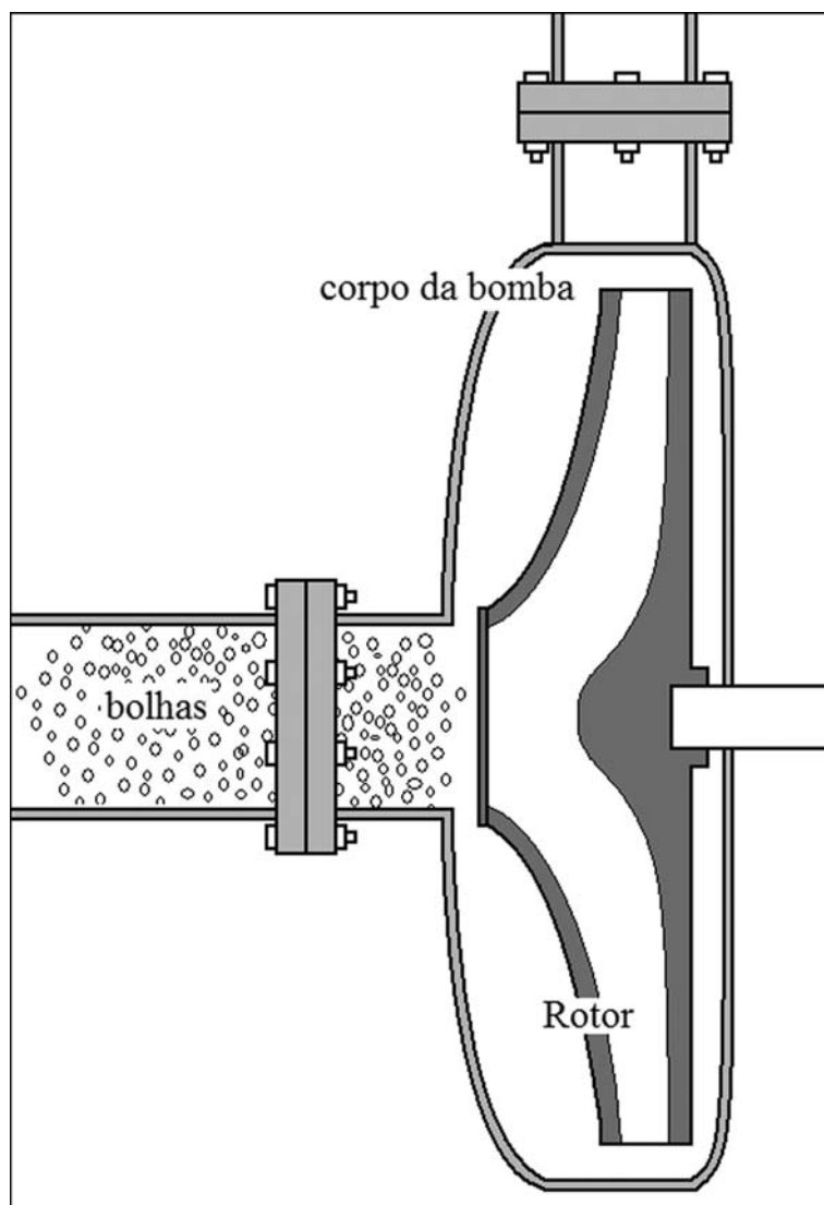
Figura 72. Cavitação.
